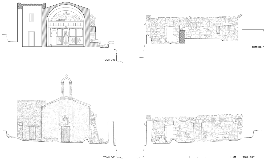
Εικ. 17. Εγκάρσιες τομές.
