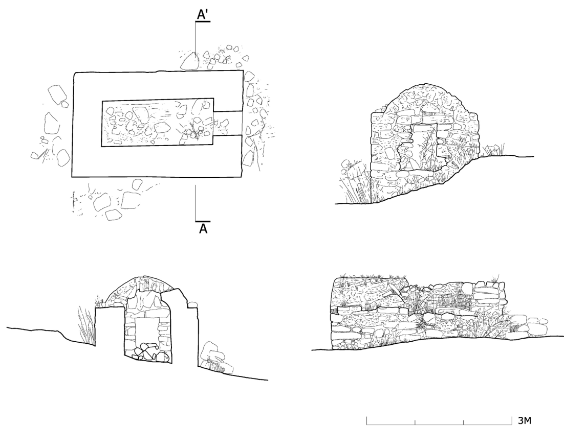
Εικ. 14. Κάτοψη, εγκάρσια τομή, ανατολική και βόρεια όψη του ταφικού μνημείου.
