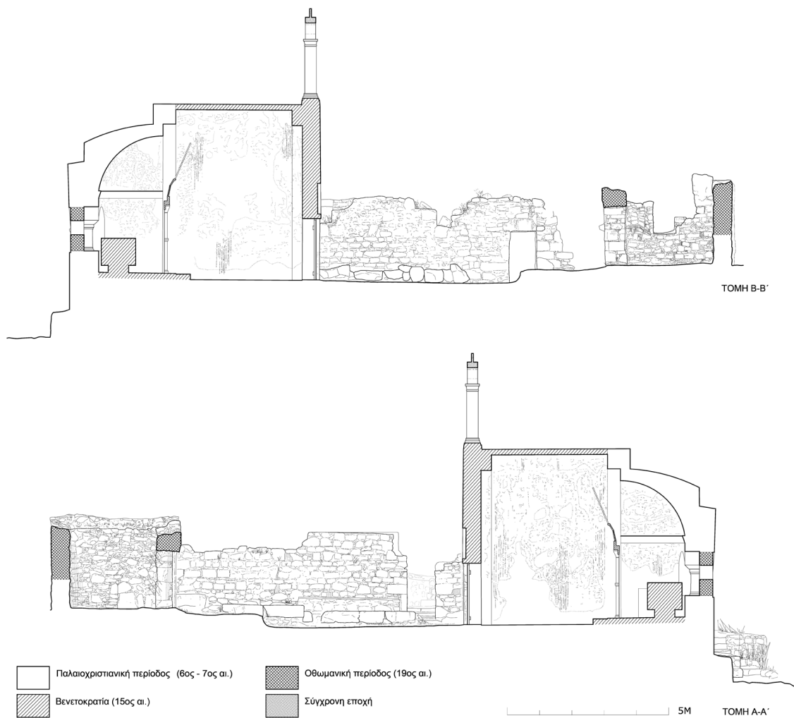
Εικ. 13. Διαμήκεις τομές.
