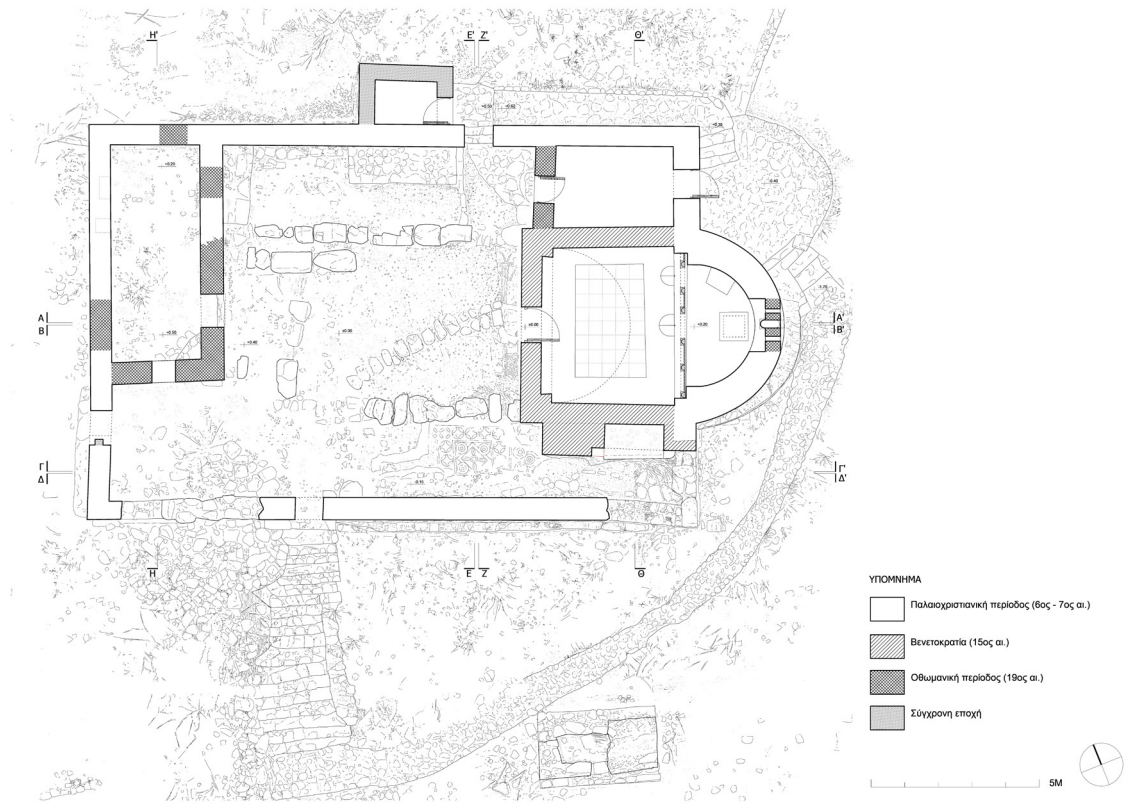
Εικ. 2. Κάτοψη.
