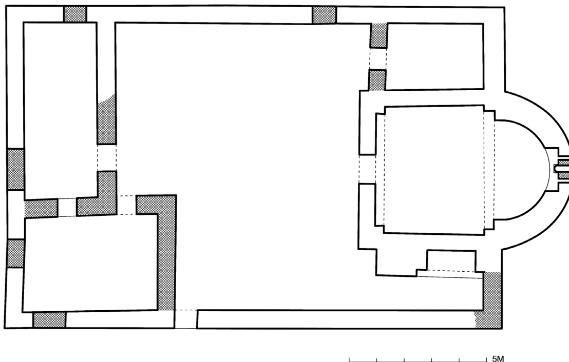
Εικ. 18. Κάτοψη του συγκροτήματος με τα τμήματα που τοιχίστηκαν κατά τον 19ο αιώνα.
