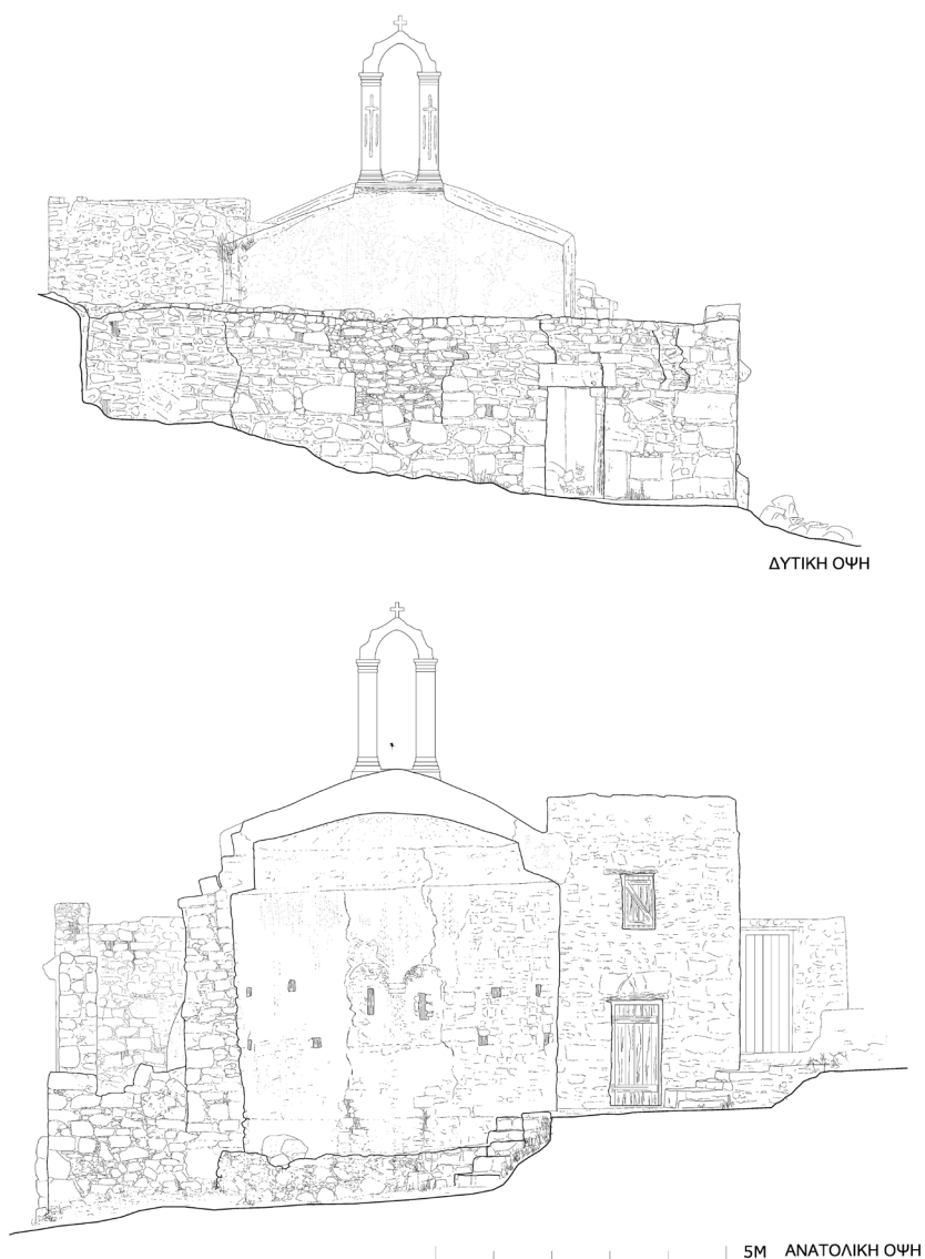
Εικ. 5. Δυτική και ανατολική όψη.
