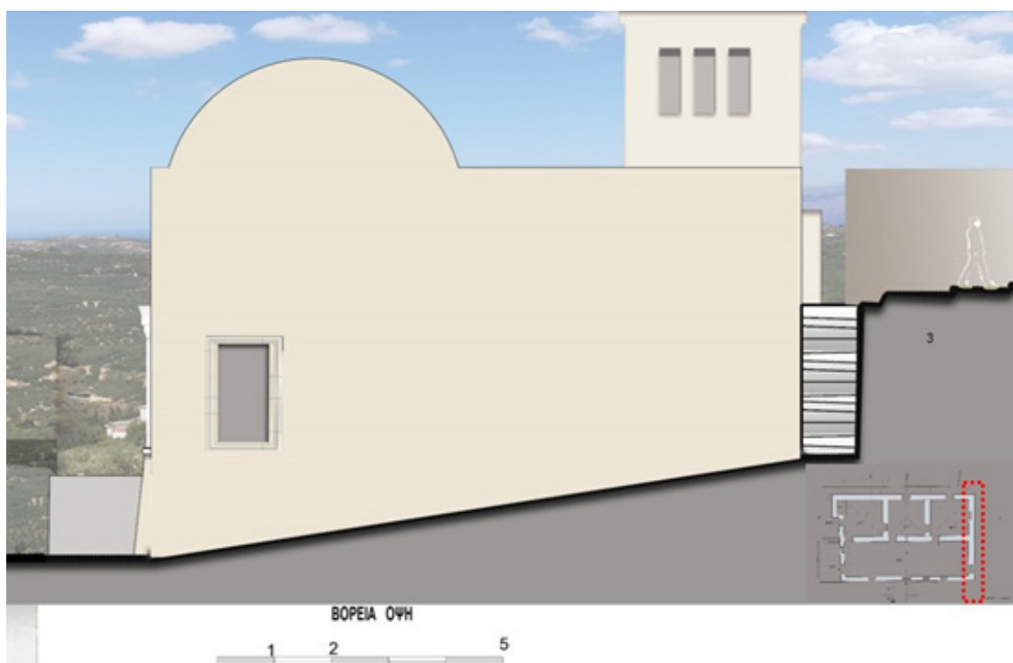
Εικ. 13. Η πιθανή βόρεια όψη του κτίσματος.
