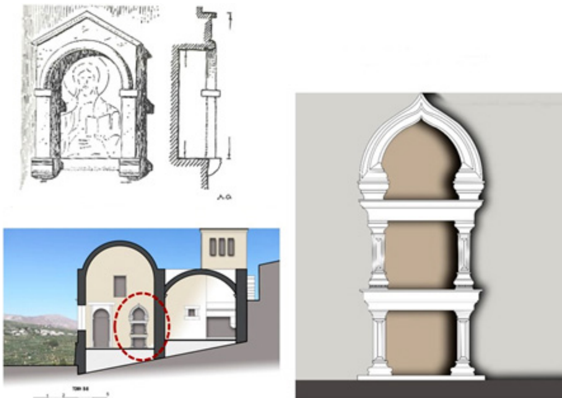
Εικ. 17. Η υπάρχουσα κατάσταση με την όψη από το προσκυνητάρι, η πρώτη αποτύπωσή του.
