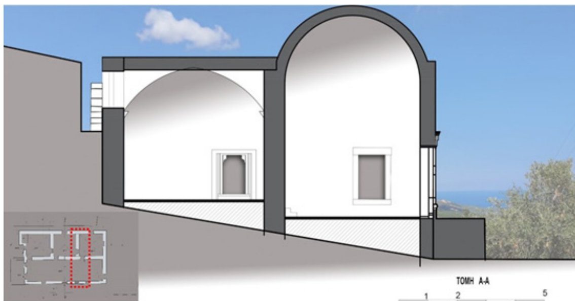
Εικ. 14. Η τομή του κτίσματος με το εσωτερικό θύρωμα και το βορινό παράθυρο.
