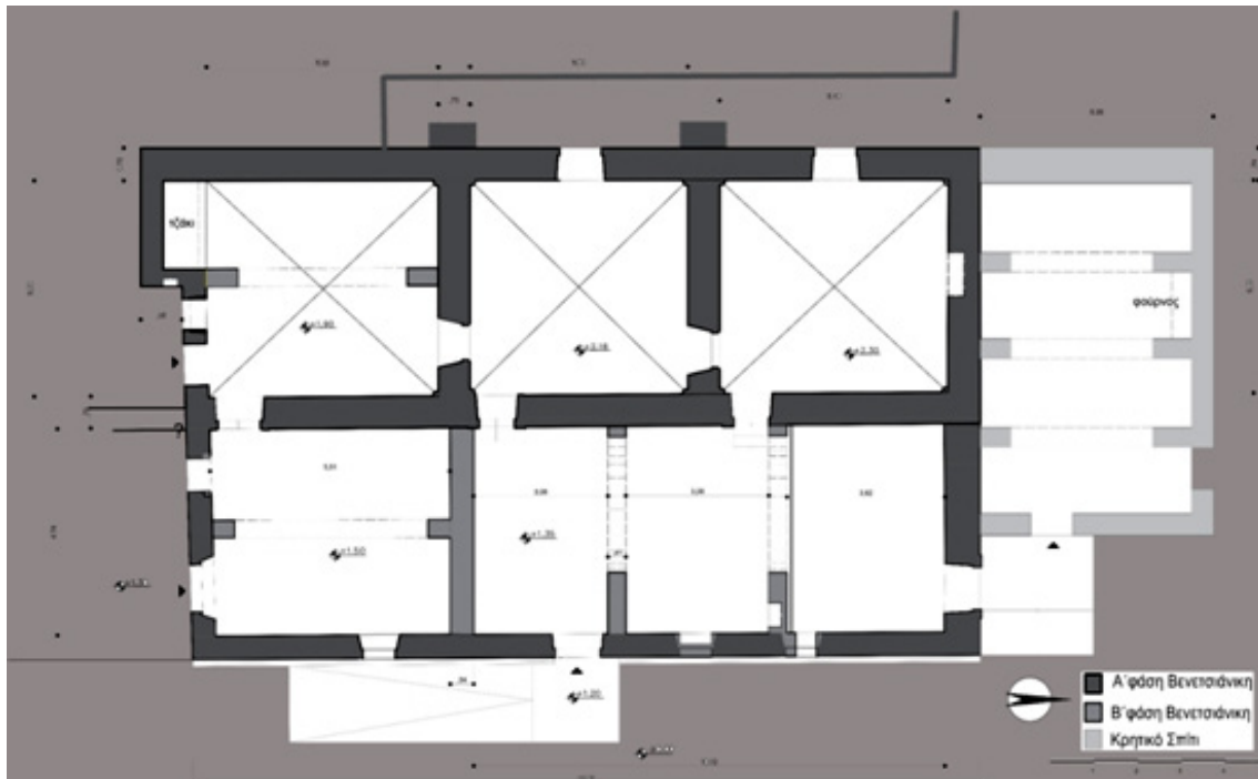
Εικ. 8. Η κάτοψη του κτίσματος με όλες τις ιστορικές οικοδομικές φάσεις επεμβάσεων.
