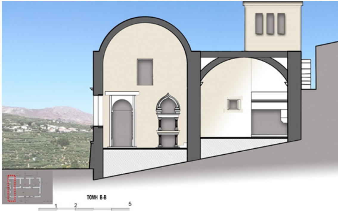
Εικ. 16. Η τομή του μεγάρου με τη μεγάλη εστία και το προσκυνητάρι μέσα στον χώρο της αίθουσας.
